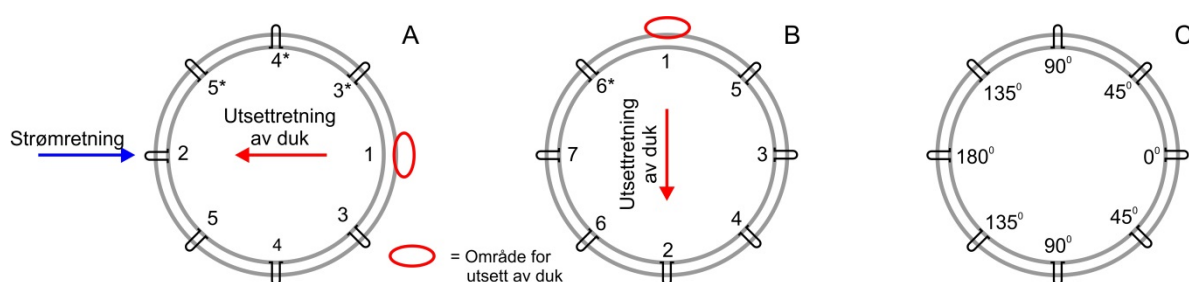
Figur 3: Utsettsretning av dukene i forhold til strøm. Nummereringen på figuren refererer til rekkefølgen hovedtauene blir dratt i. Alle lik nummererte punkter med hovedtau dras samtidig (eksempelvis 3 og 3*). A): Strømretning motstrøms, der punkt 1 er utsettspunktet for duken. Hovedtau 2 kalles her for 180° der man starter å dra mot, 3 og 3* kalles for 45°, 4 og 4* kalles for 90°, og 5 og 5* for 135°. B): Strømmen 90° på utsettretningen med utsett fra punkt 1, og der 3 er 0°, 4 og 5 er 45°, 6 og 6* er 135° og 7 er 180°. C): Viser vinklene i forhold til strømretning.
